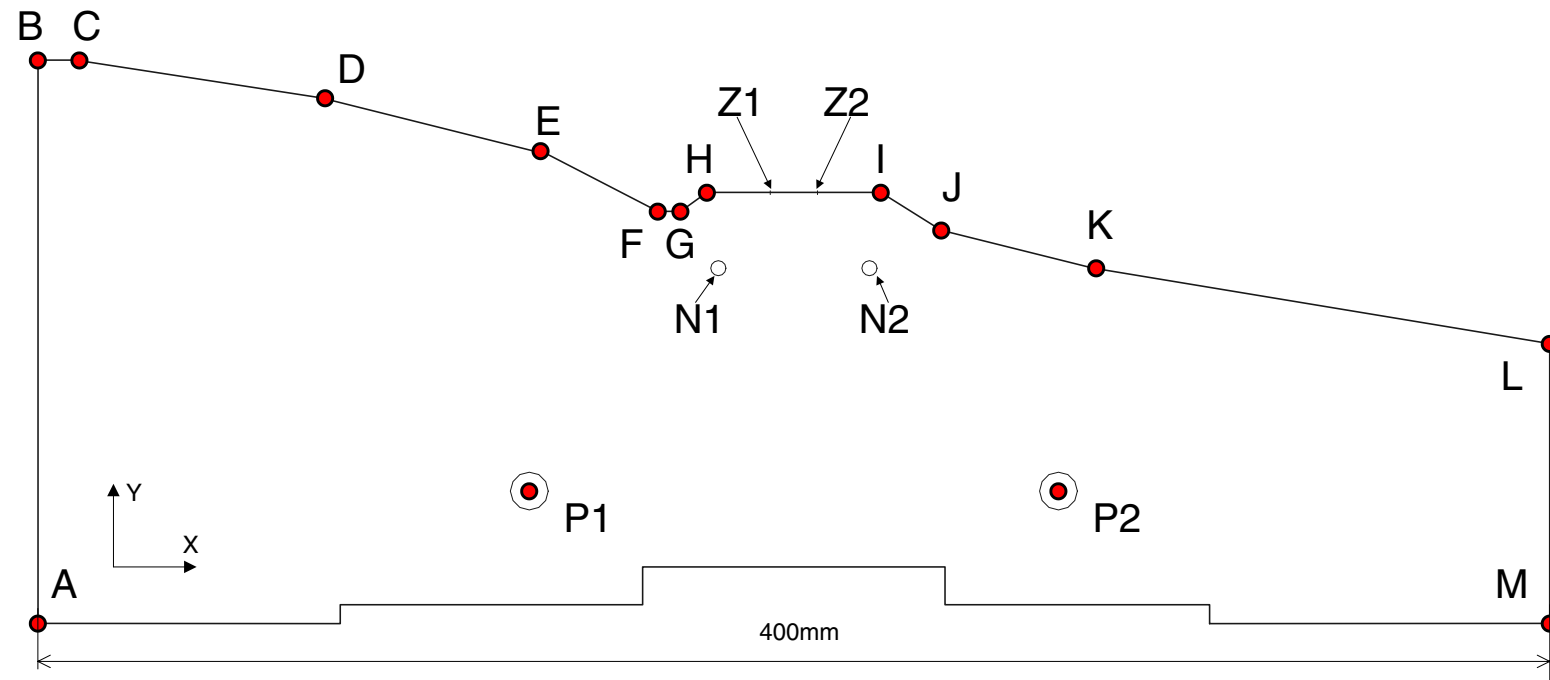
Výkres styčného profilu modulů velikosti TT (1:120), používaného v KŽM Praha 3.
